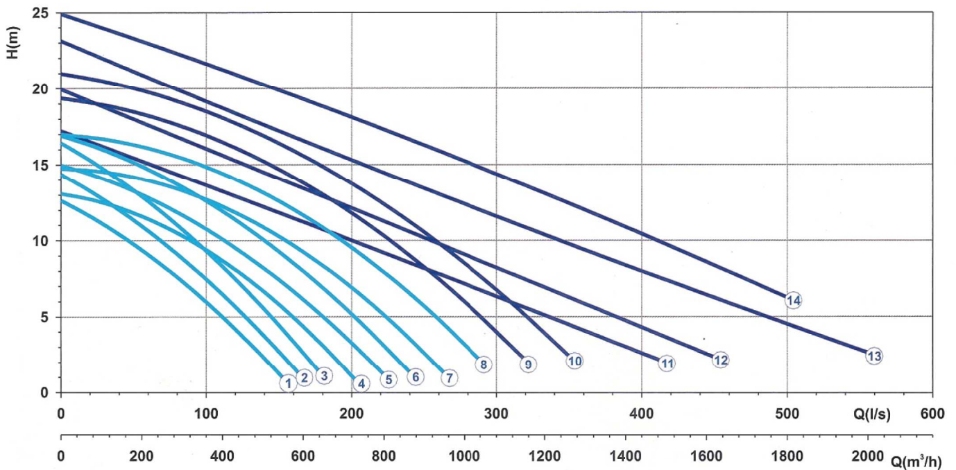
R.P.M. 950
